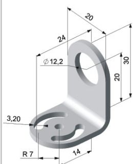
Uchwyt mocujący, stały
