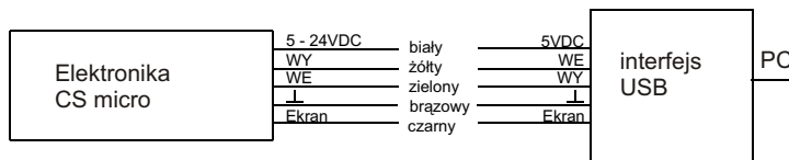
Schemat podłączenia pirometr CSmicro – interfejs USB
